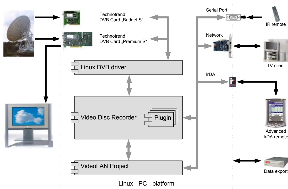
Abbildung 2.3.: Struktur des Digitalen Video Projekts
