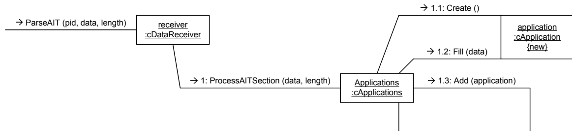
Abbildung 4.19.: Funktionsweise des AIT-Parsers
